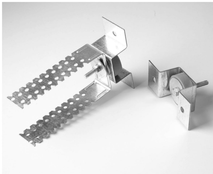
Крепления Vibrofix P и Vibrofix PU
