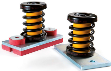
Vibrofix Spring DSD
