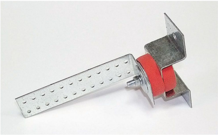
Vibrofix Uni L
