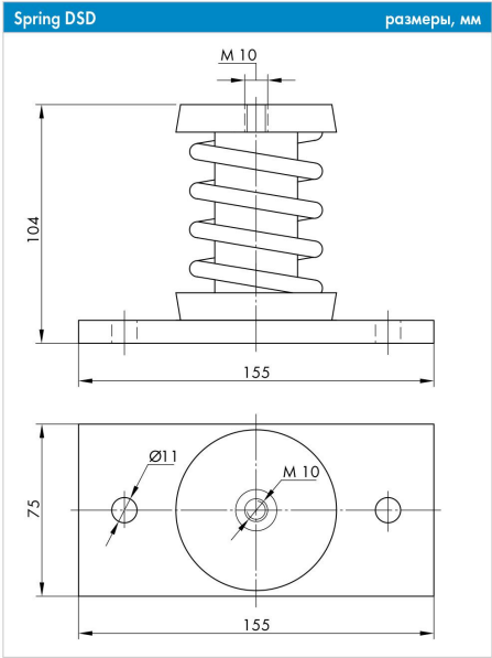
Vibrofix Spring DSD
