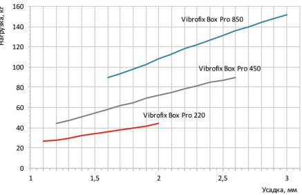
Усадка упругого элемента в зависимости от нагрузки на крепление
