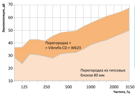
Звукоизоляция перегородки из гипсовых блоков (воздушный шум):
